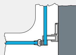
Detal A - widok z góry
