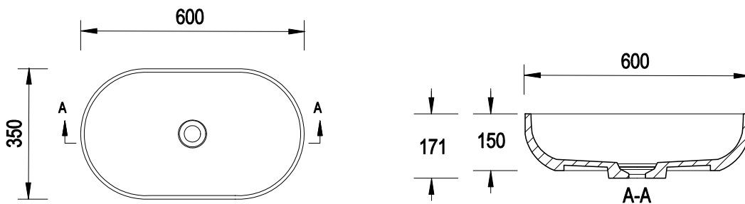
FIRA 60x35x17,1 cm (EMPORIA-FIRA0002)
