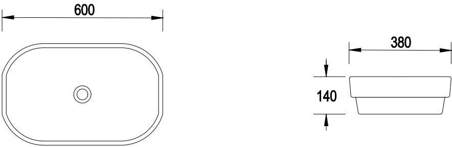
EGIA 01 60x38x14 cm (EMPORIA-8540)
