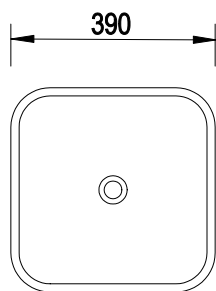
BARI 01 39x39x13 cm (EMPORIA-LT-2196)
