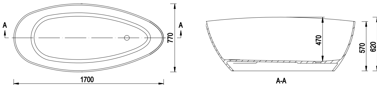
RIVA 170x77x57 cm (EMPORIA-RIVA0002)
