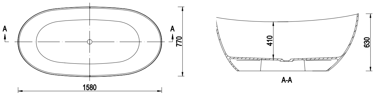
LUNA 158x77x63 cm (EMPORIA-LUNA0001)
