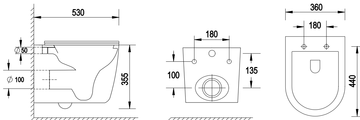
NOX 2.0 53x36x35,5 cm (EMPORIA-ABD002)
