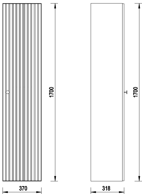
RIO 37 37x31,8x170 cm (EMPORIA-001-C-03702 | EMPORIA-001-C-03703)
