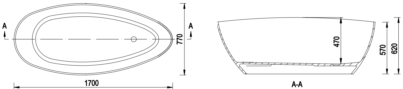
RIVA 170x77x57 cm (EMPORIA-RIVA0002)
