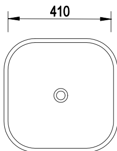
FIBI 01 41x41x15 cm (EMPORIA-LT-2144)
