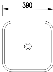
BARI 01 39x39x13 cm (EMPORIA-LT-2196)
