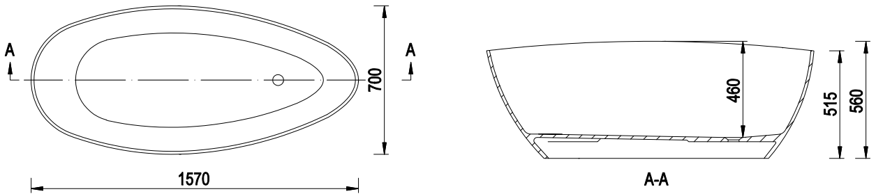
RIVA 157x70x56 cm (EMPORIA-RIVA0001)
