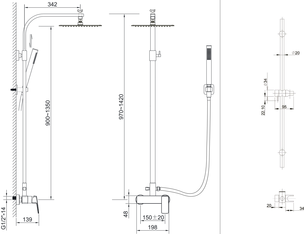
EMPORIA-020110 Kolumna natryskowa
