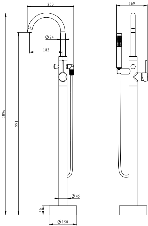
EMPORIA-03031 Batera wannowa
