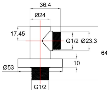
EMPORIA-04085 Przylécze kątowe
