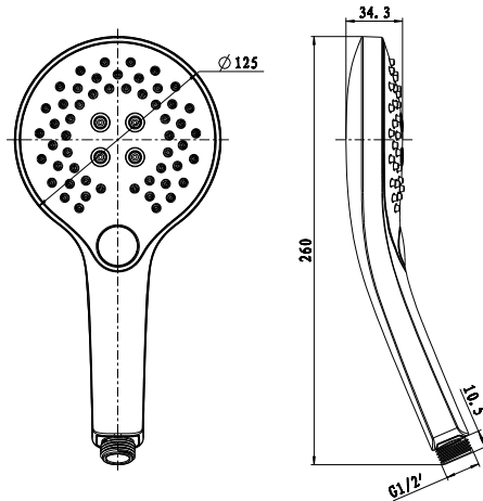
EMPORIA-040731 Słuchawka prysznicowa
