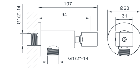
EMPORIA-04080 Przylécze kątowe
