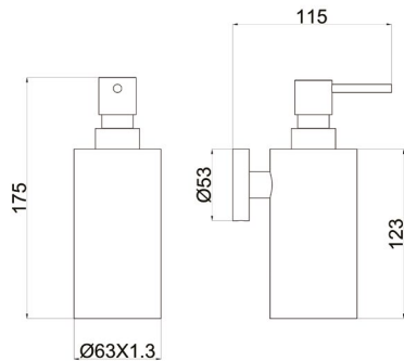
EMPORIA-5070 Dozownik na mydło
