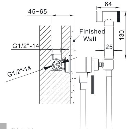
EMPORIA-01021 Bidetta ścienna
