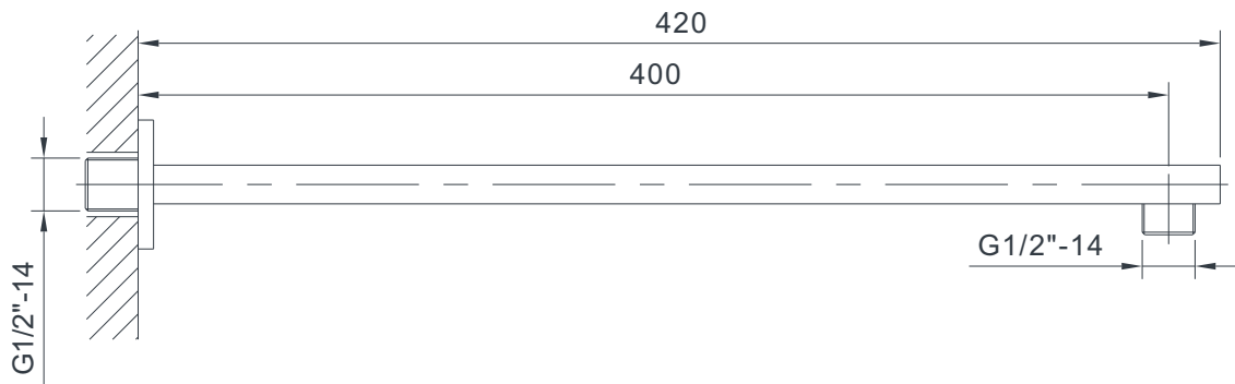
EMPORIA-04051 Ramię deszczownicy
