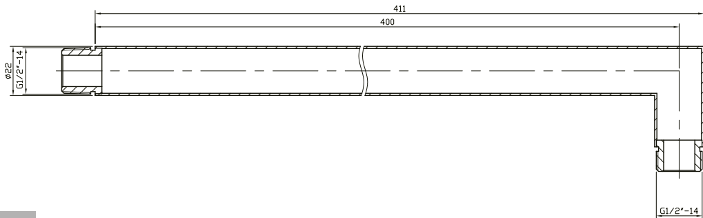
EMPORIA-04050 Ramię deszczownicy
