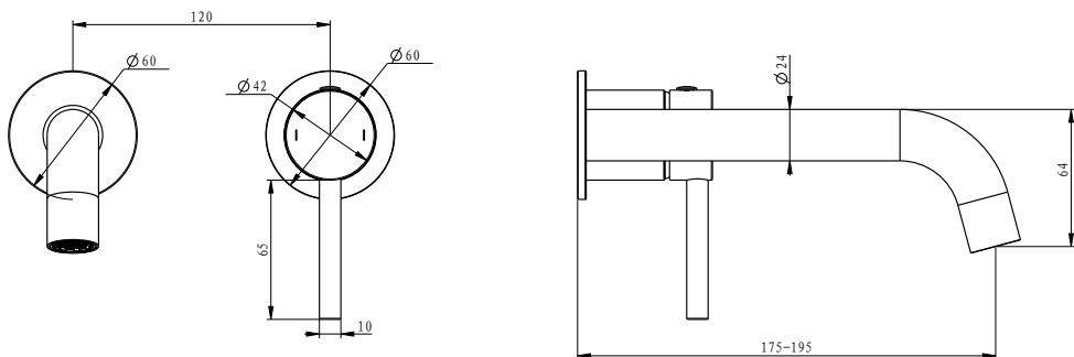
EMPORIA-03012 Bateria umywalkowa
