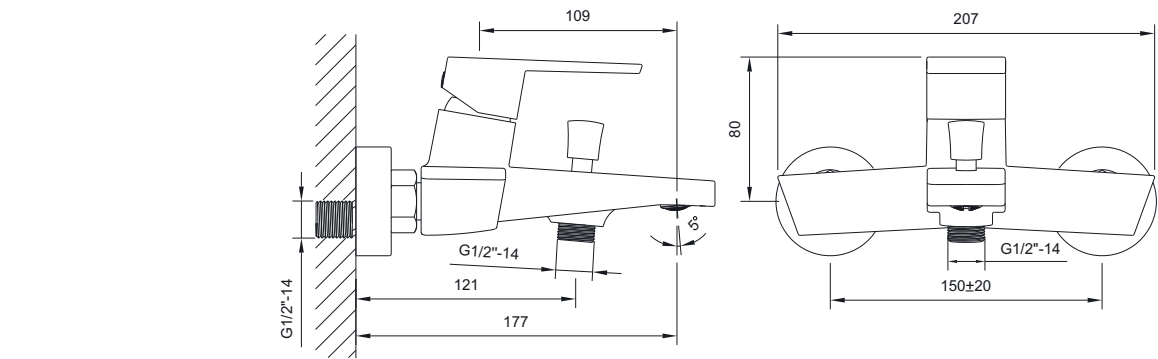
EMPORIA-02030 Bateria wannowa
