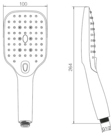
EMPORIA-040732 Słuchawka prysznicowa
