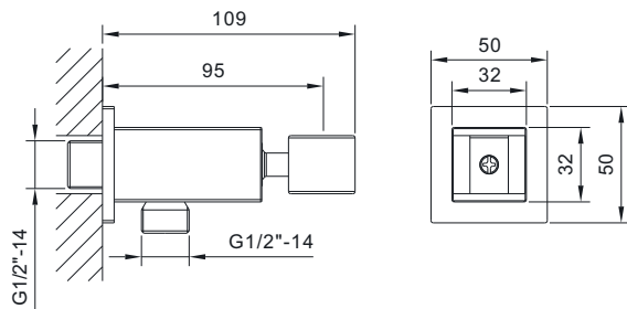
EMPORIA-04081 Przyłtęcze kątowe
