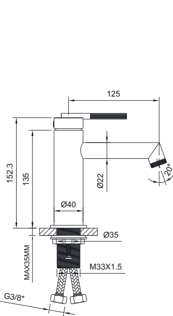
EMPORIA-01010 Bateria umywalkowa
