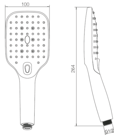
EMPORIA-040732 Słuchawka prysznicowa
