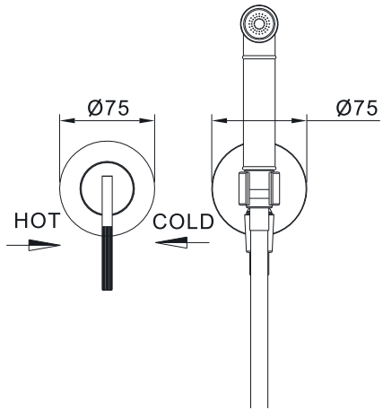
EMPORIA-01020 Bateria bidetowa
