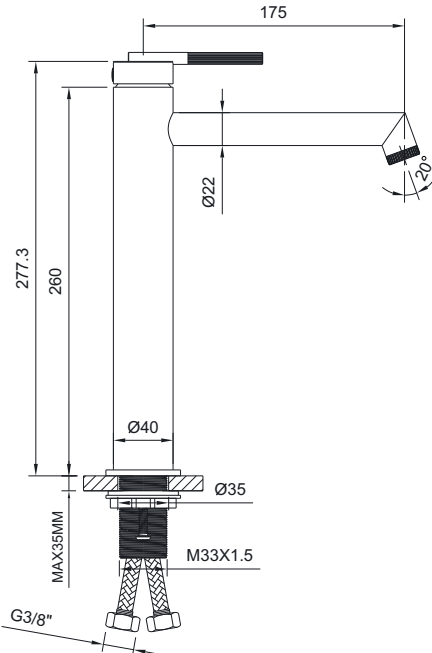
EMPORIA-01011 Bateria umywalkowa
