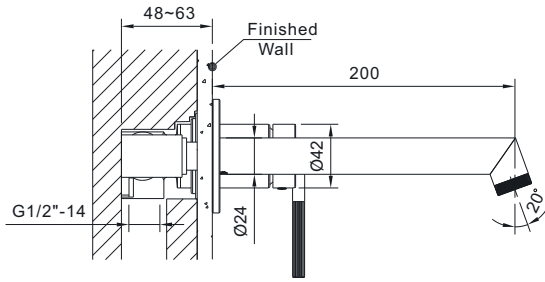
EMPORIA-01012 Bateria umywalkowa
