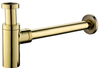
Syfon umywalkowy okrągły, regulowany, przyłącze 1 1/4, odpływ 32 mm, złoty EMPORIA-HF6009-G
