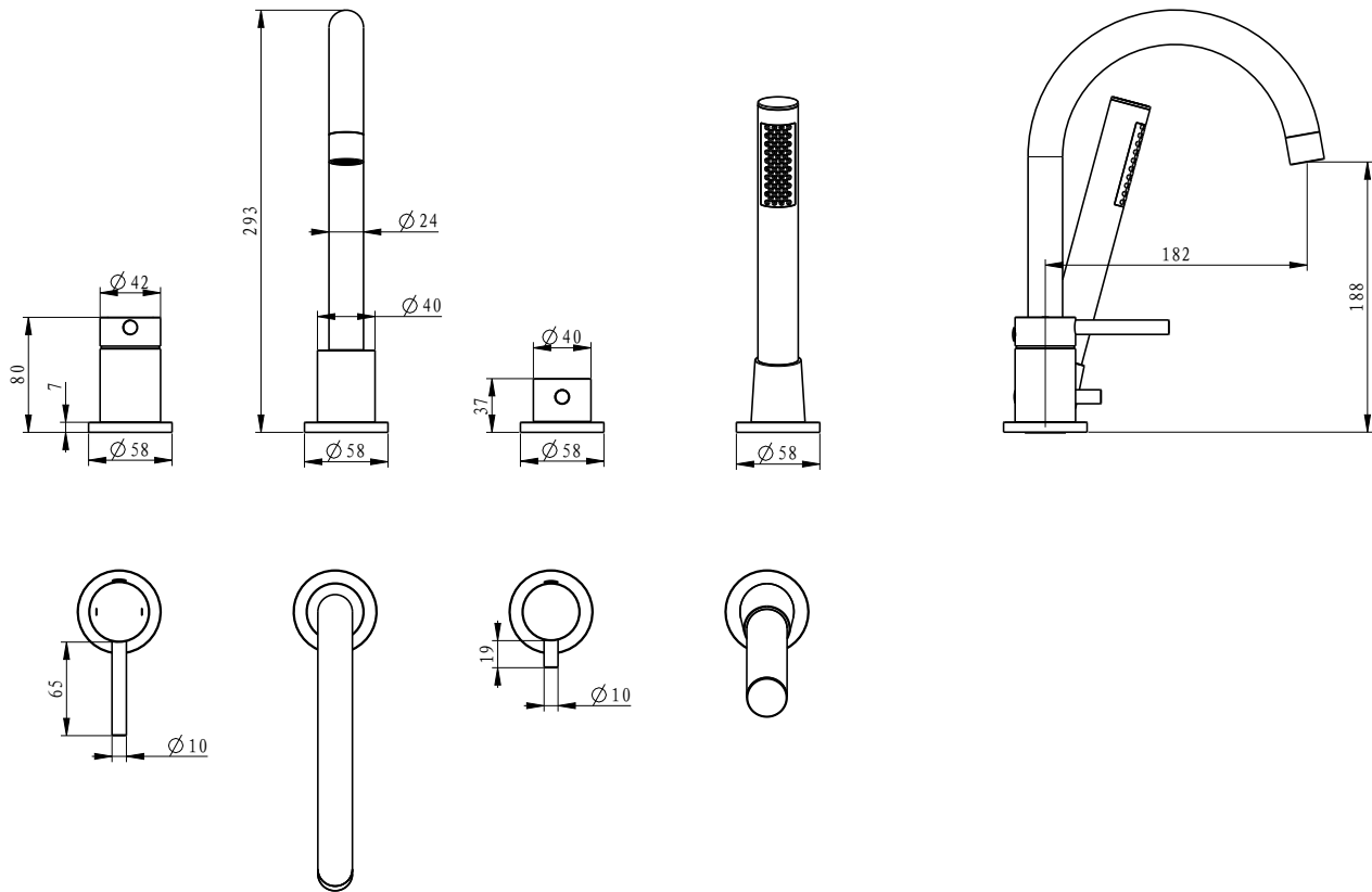
EMPORIA-03033 Bateria wannowa
