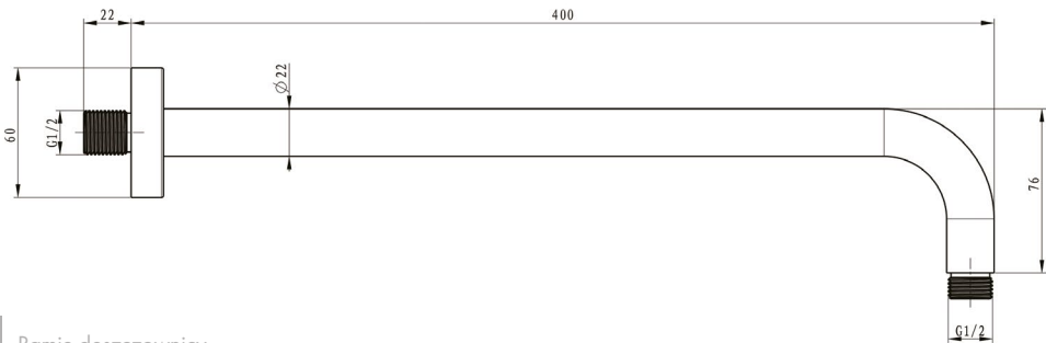
EMPORIA-04052 Ramię deszczownicy
