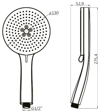
EMPORIA-040733 Słuchawka prysznicowa
