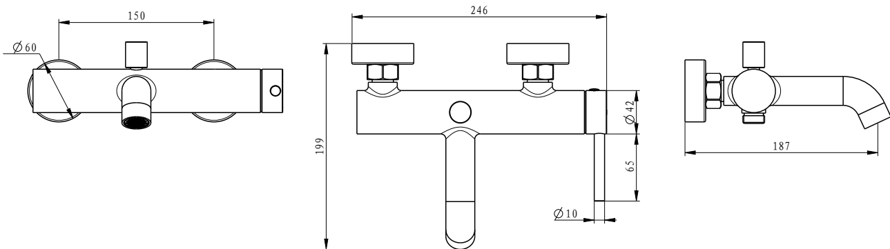
MPORIA-03030 Bateria wannowa
