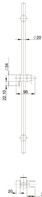
EMPORIA-040180 Drążek prysznicowy
