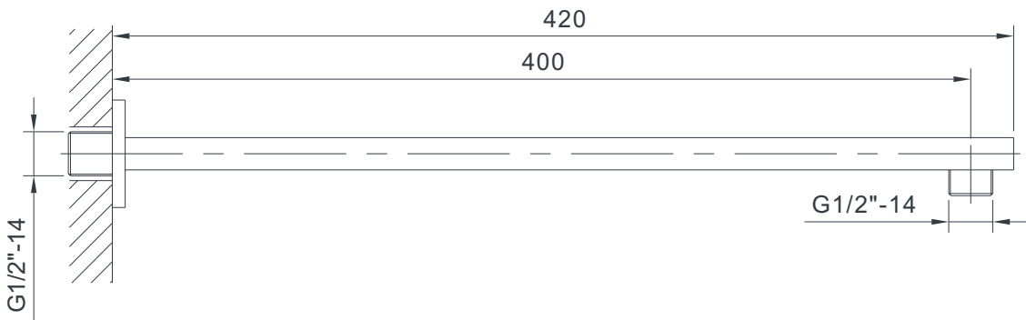
EMPORIA-04051 Shower arm
